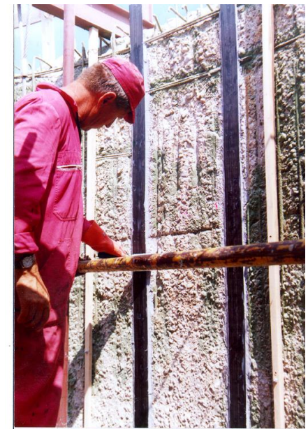
Plašč hladilnega stolpa TE Šoštanj - (prva aplikacija dolepljene kompozitne armature v Sloveniji) 1996
