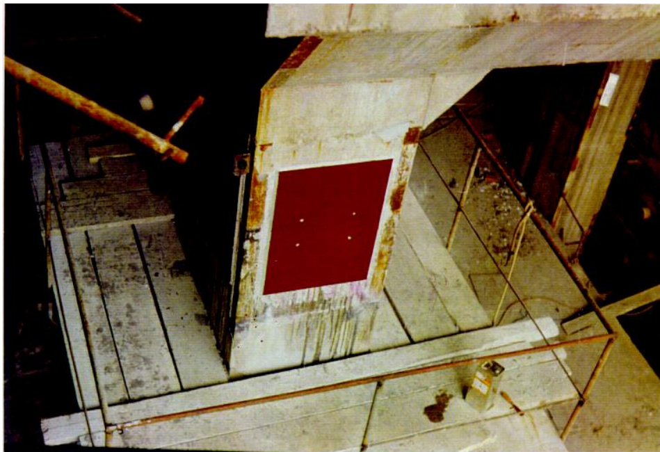
Delovni stiki stebrov temelja 230 MW agregata TE Kakanj, BIH (1985)
