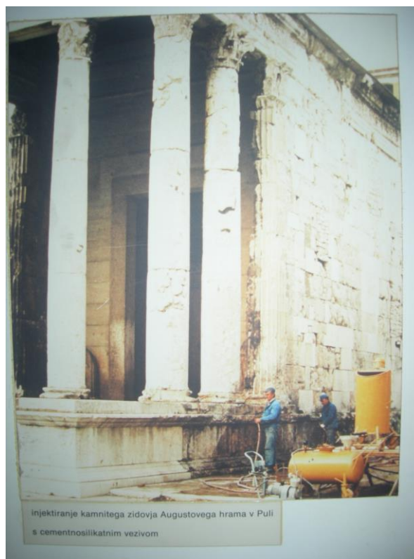
SANACIJA AVGUSTOVEGA HRAMA, PULA, HRVAŠKA
